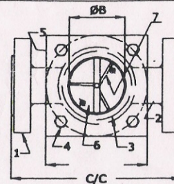
ROTOR
