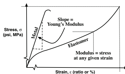
Tensile, elongation, modulus
